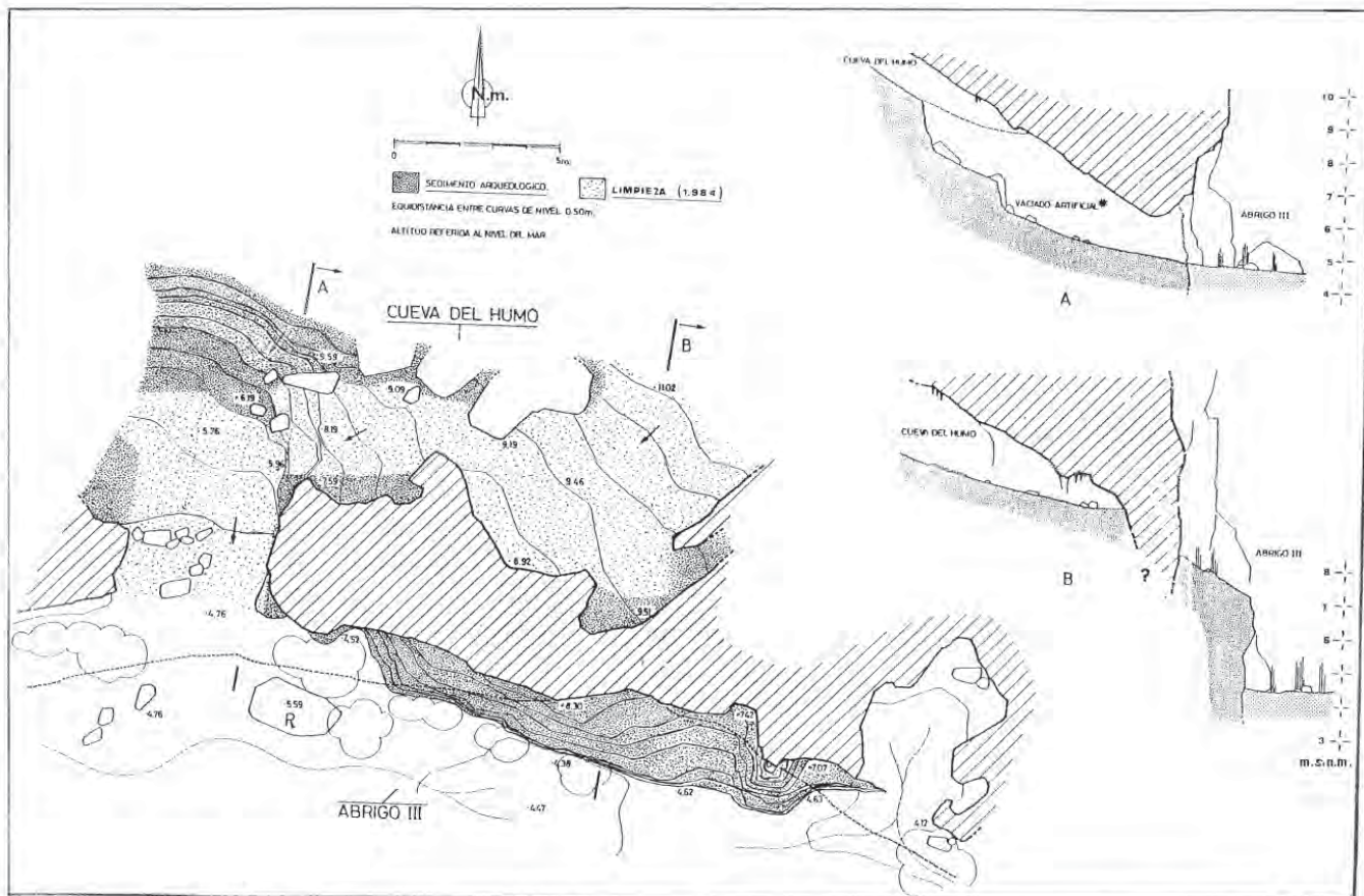
FIG. 3. Plano de la entrada de la Cueva del Humo y secciones de entrada (A) y de la Sala del Abrigo (B).
